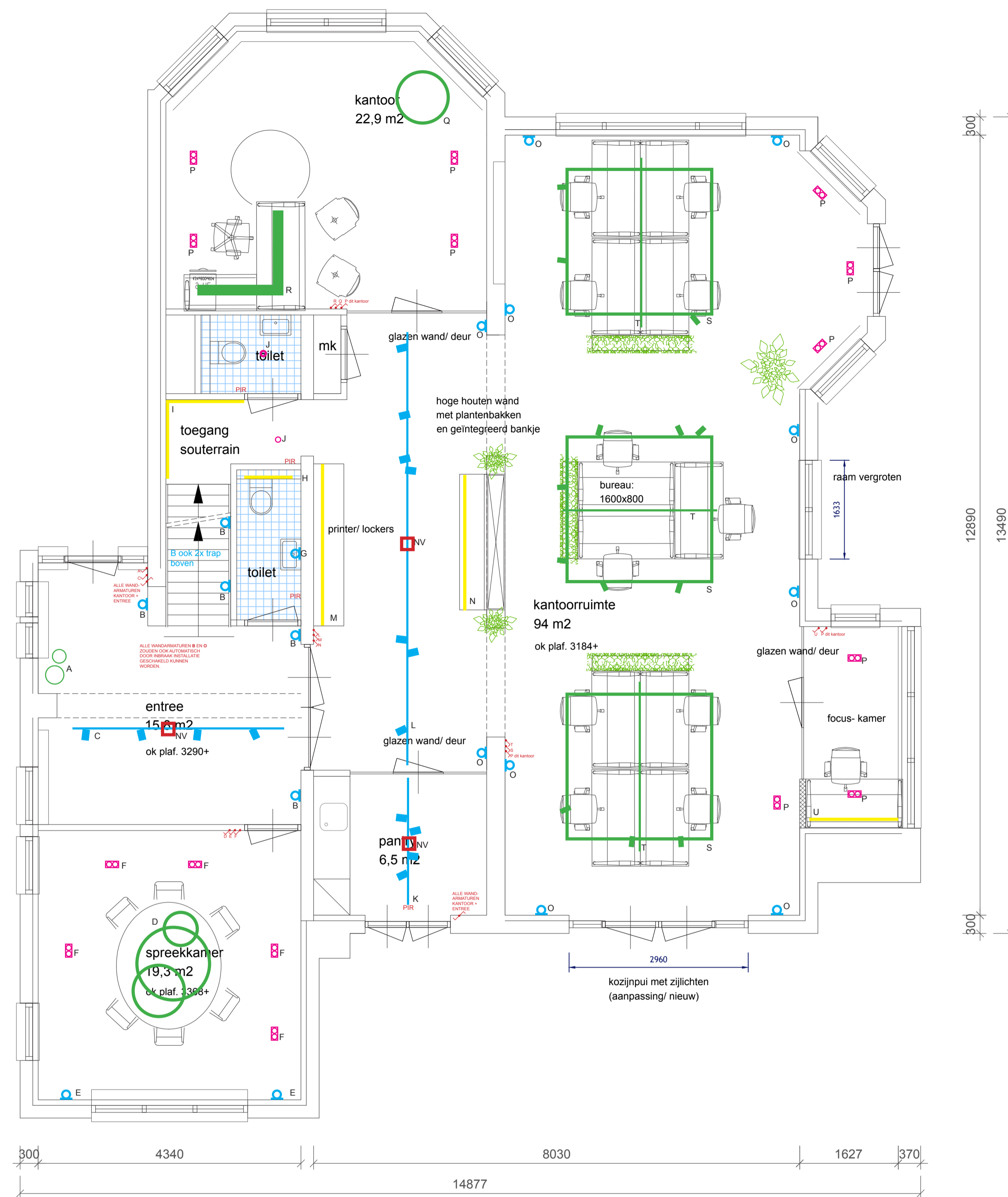
begane grond C. nieuwe situatie
